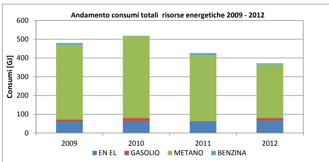
Grafico 1 - Andamento consumi totali risorse energetiche nel periodo 2009 – 2012
